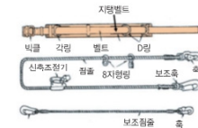
[ U자걸이용 안전대 ]
